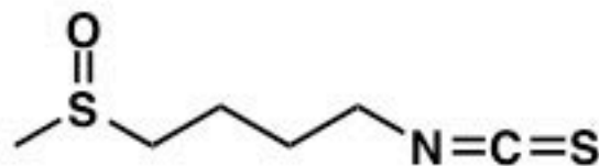
Sulforaphane (SFN)
