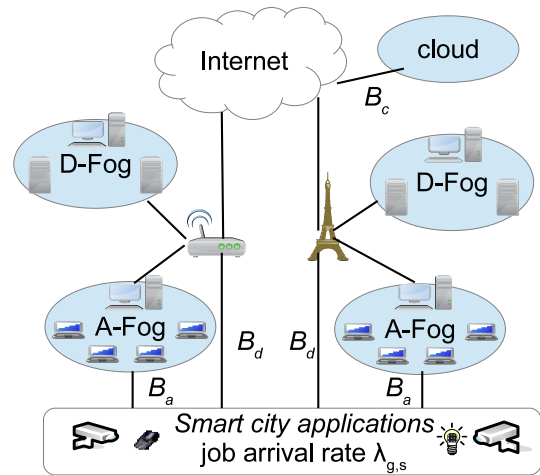
Fig. 6. Fog system scenario.
